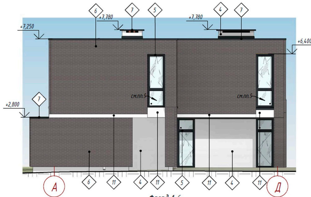
Фасад 1-6
