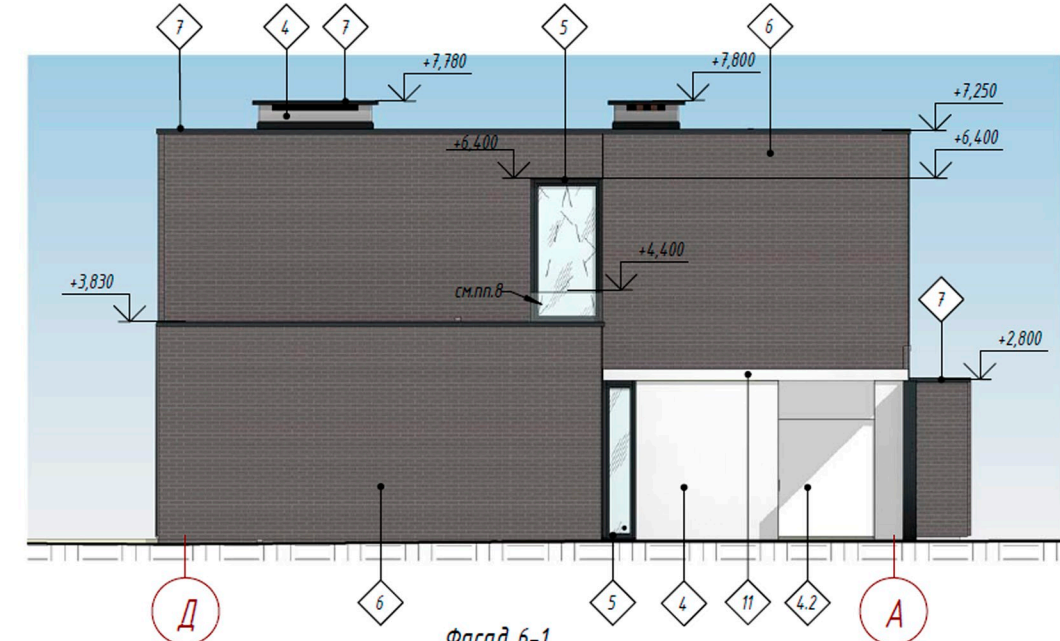
Фасад 6-1
