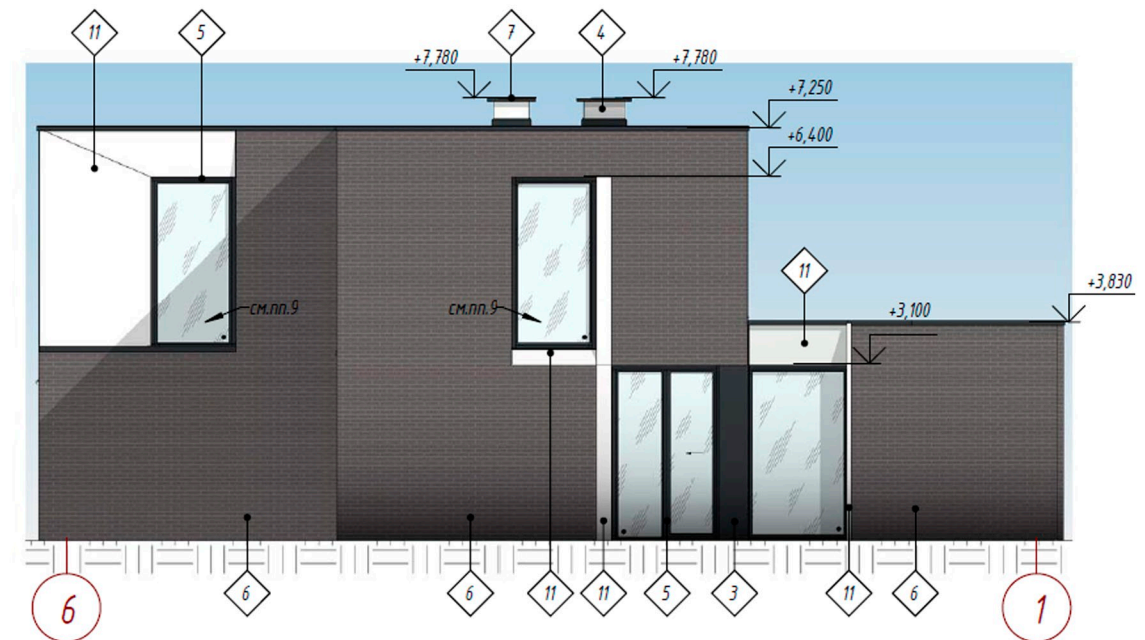
Фасад 6-1
