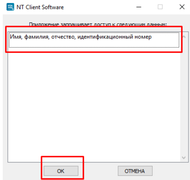
Рисунок 3. Окно КП
